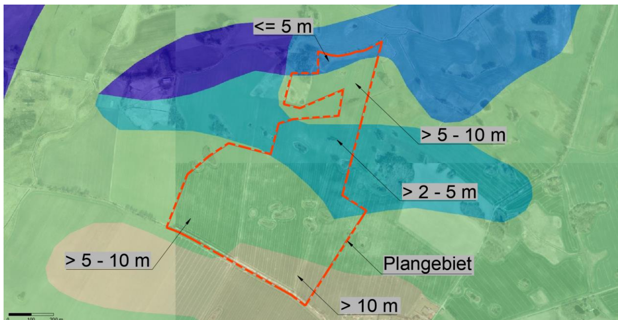
Abb. 8: Grundwasserflurabstände (© GeoBasis-DE/M-V 2023)
